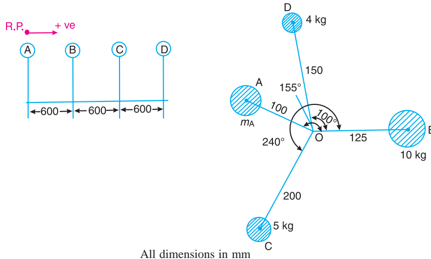
(a) Position of planes. (b) Angular position of masses. (c) Couple polygon. (d) Force polygon.
