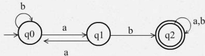
Fig. 1. A DFA
